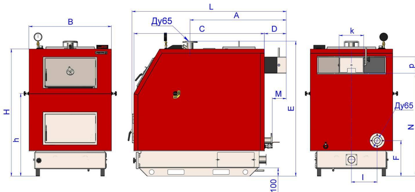
Рис.2 Котли модельного ряду «Петра-3М»
