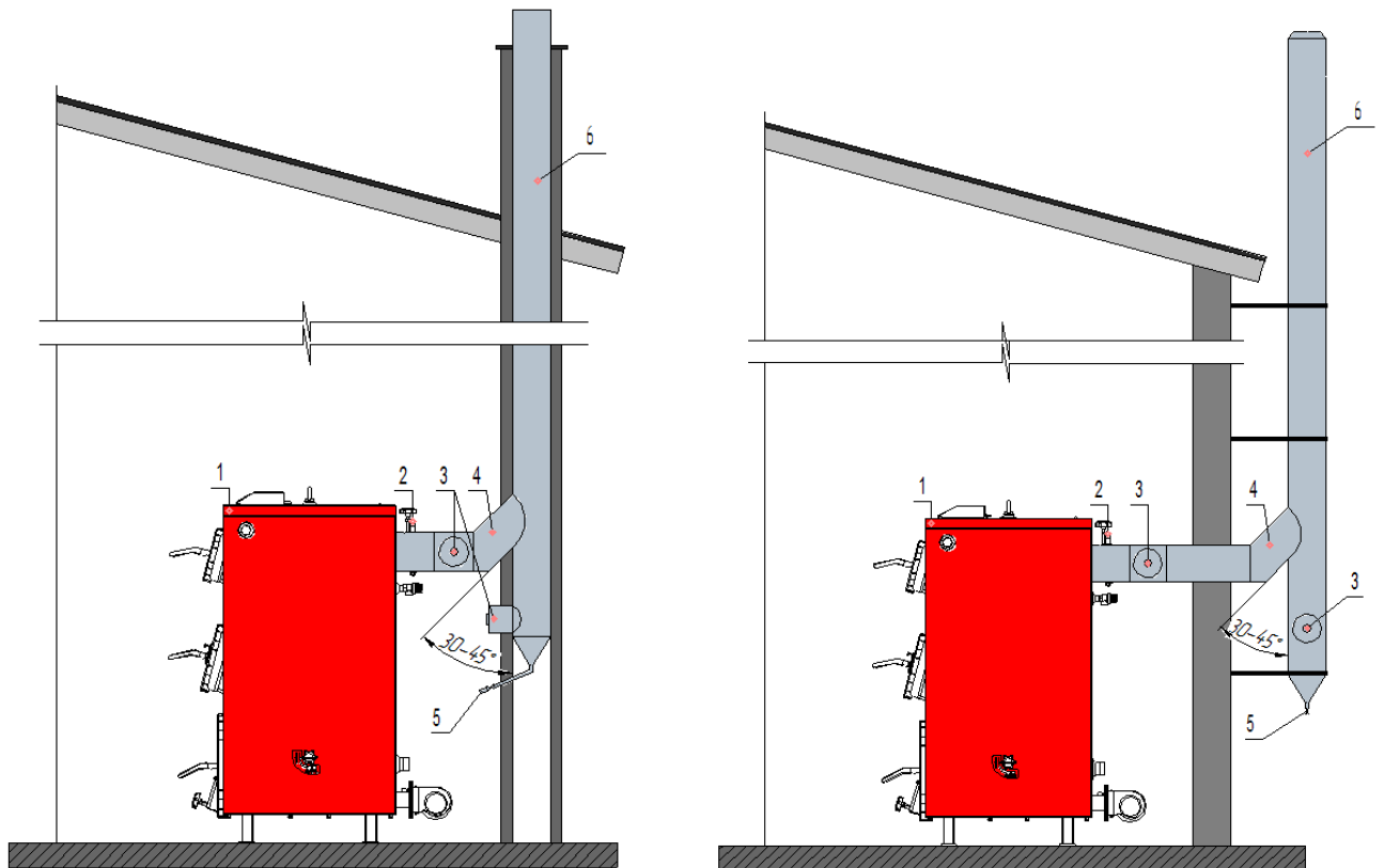
Рис.8 Рекомендована схема по під'єднанню котла до димоходу
